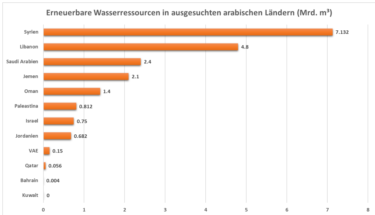
Abbildung 5.1: Erneuerbare Wasserressourcen in ausgewählten arabischen Ländern (Mrd. m 3 ), Quelle[2]
