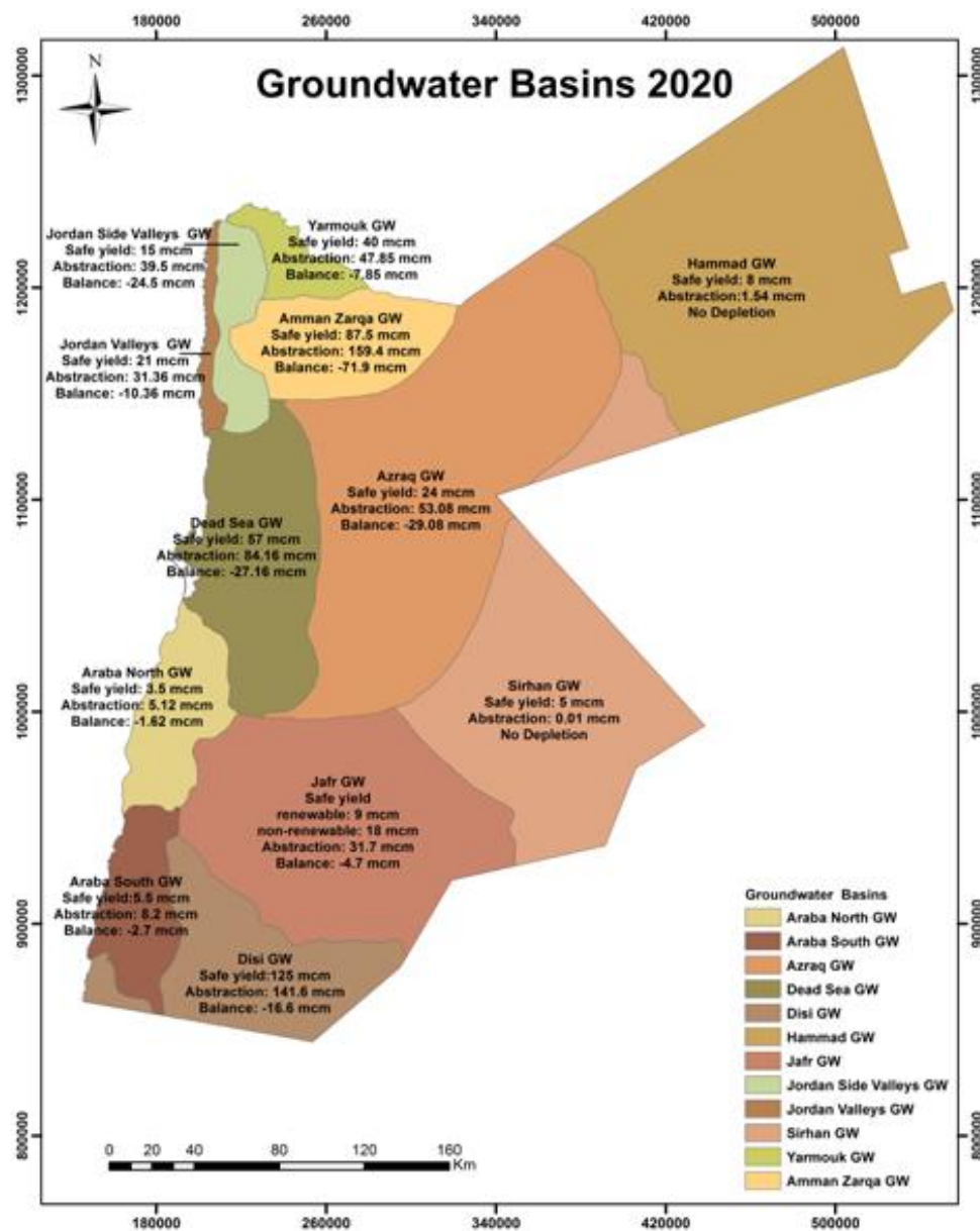
Abbildung 5.3: Karte der Grundwassereinzugsgebiete, Quelle: [4]
