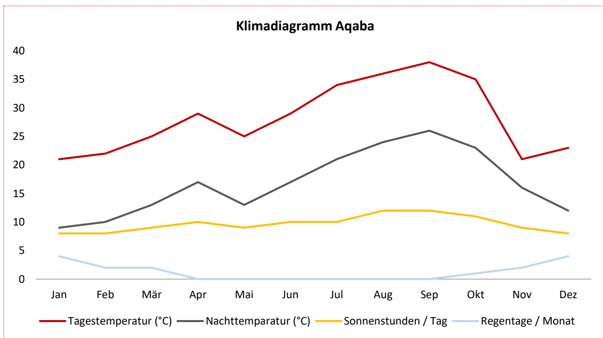
Abbildung 3.3: Klimadiagramme Amman und Aqaba
