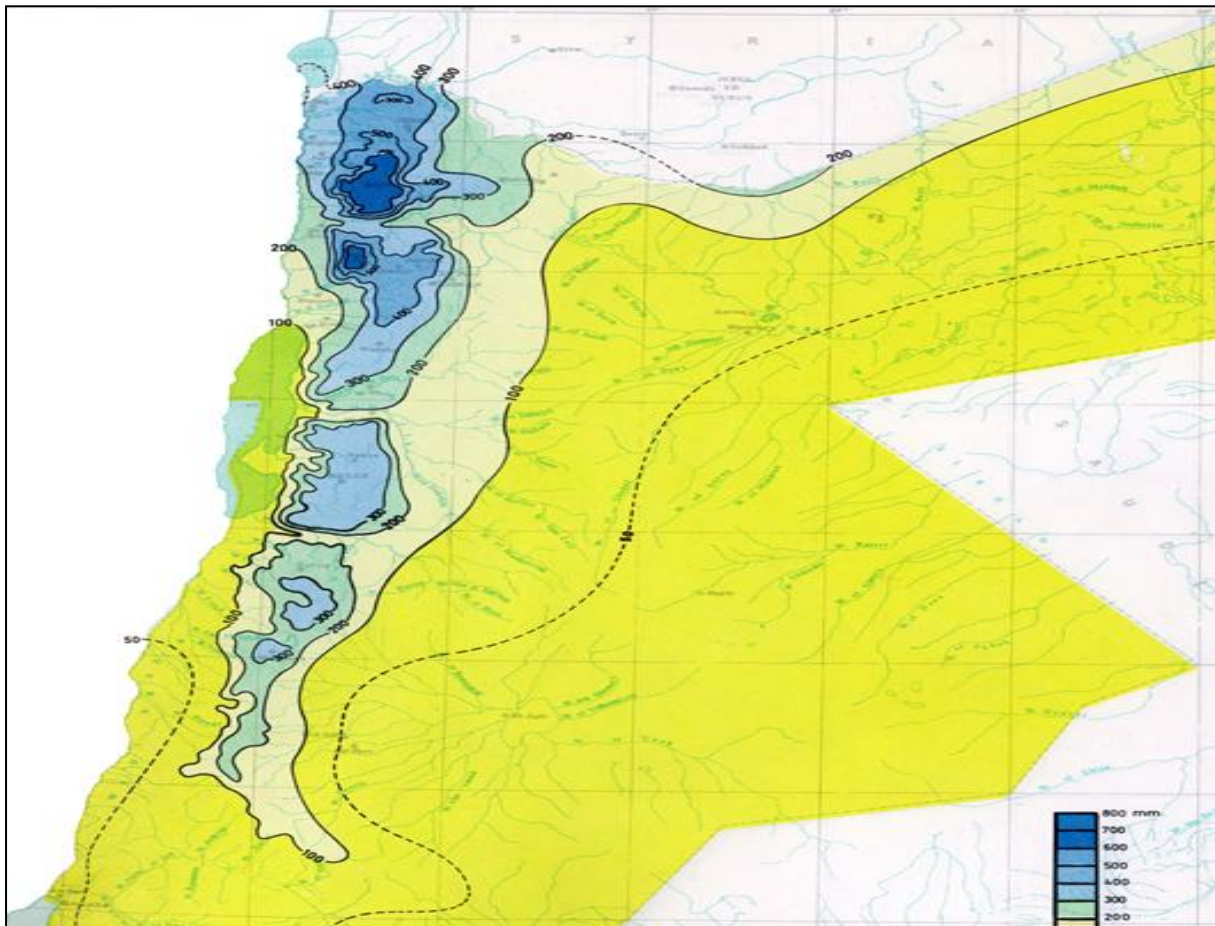
Abbildung 3.4: Karte Niederschlag Jordanien
